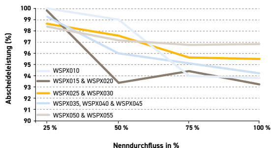
OIL-X Klasse WS Wasserabscheider Effizienz Flüssigkeitsabscheidung (25 - 100 % Nenndurchfluss)
