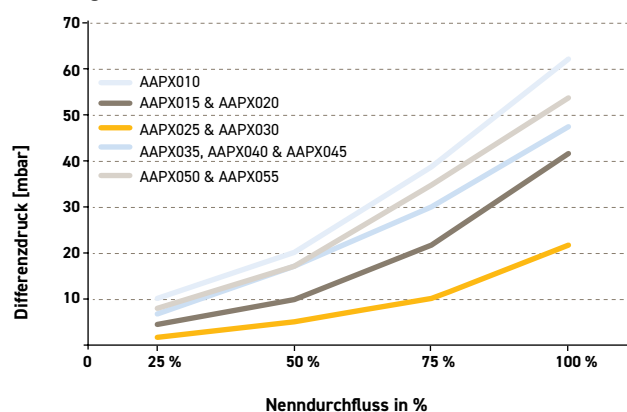
OIL-X Klasse AA Trockenpartikelfilter Anfänglicher Differenzdruck (trocken) (25 - 100 % Durchflussrate)
