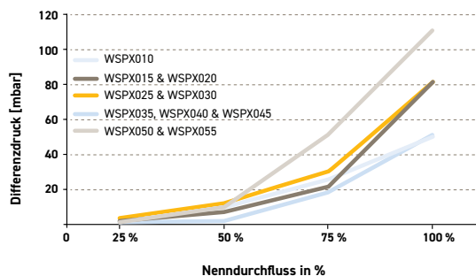
OIL-X Klasse WS Wasserabscheider Differenzdruck (25 - 100 % Nenndurchfluss)
