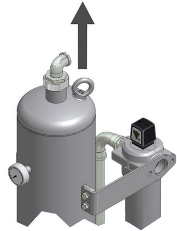
Transportöse am Druckbehälter
