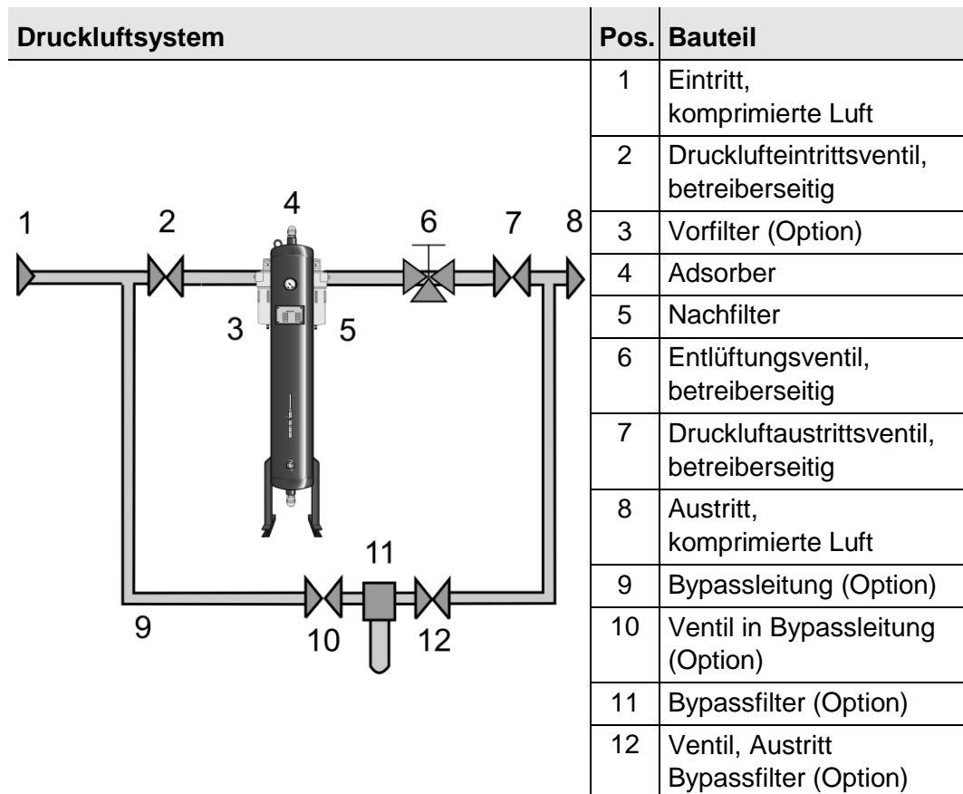
Beispiel einer Installation mit Bypassleitung
