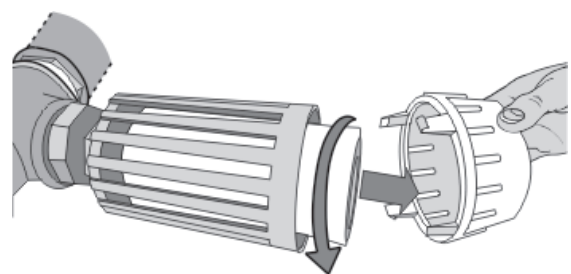
Schalldämpferelement erneuern
